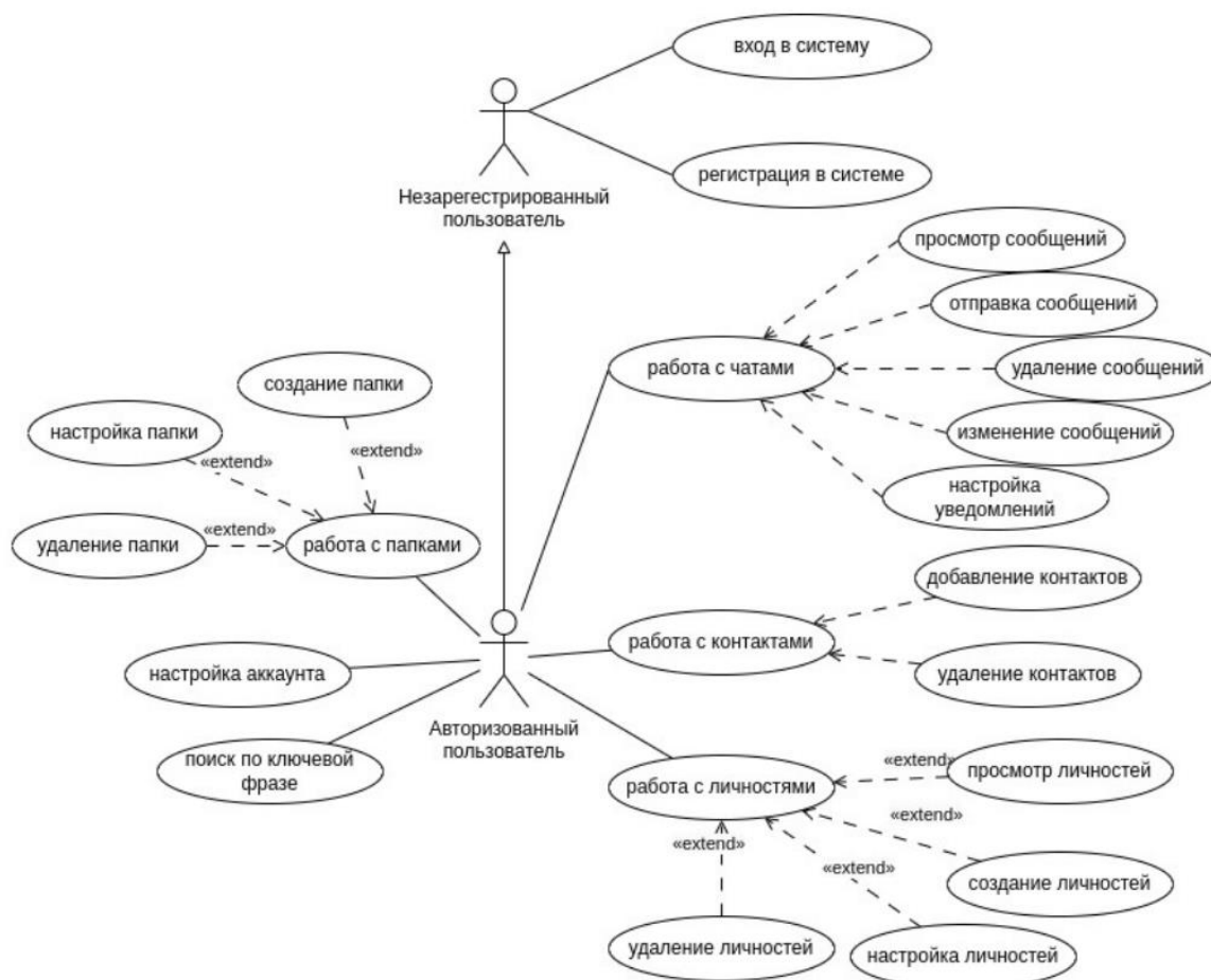
Рис. 1. Функции мессенджера с разделением сфер общения
