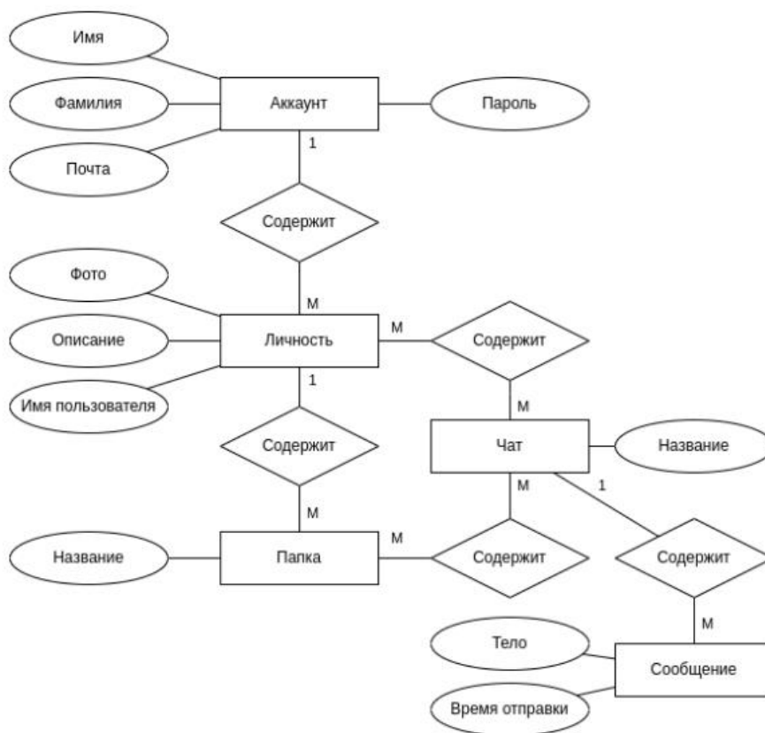
Рис. 2. Фрагмент схемы базы данных для хранения информации о личности пользователя
