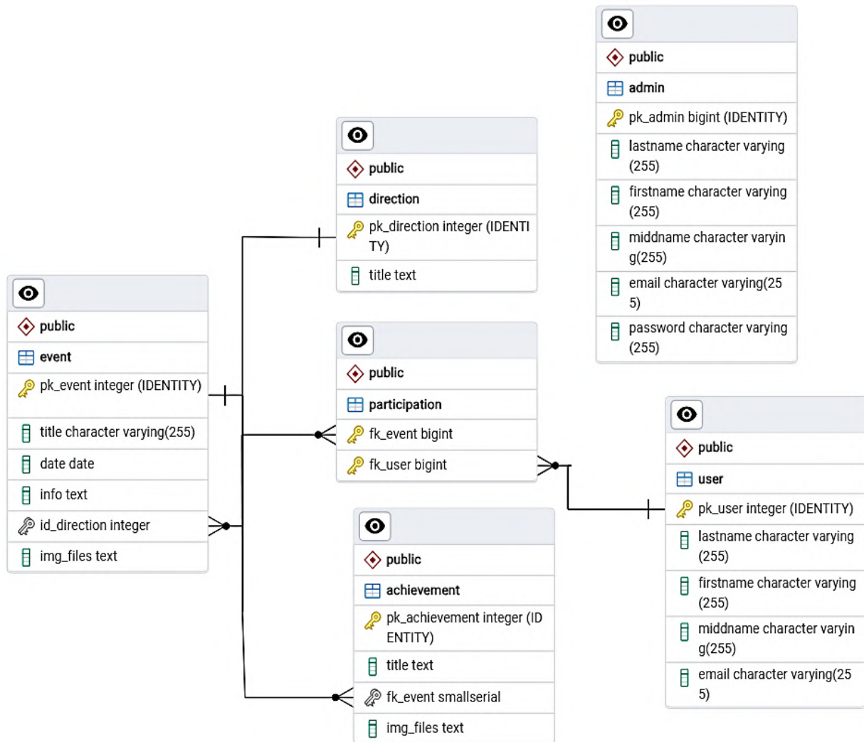
Рис. 2. Схема БД
