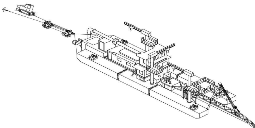
Рис. 2. Схема вытаскивания земснаряда из воды
