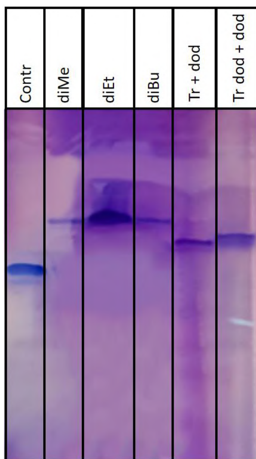
Рис. 20. Электрофорез в денатурирующих условиях в 20% ПААГ с соотношением акриламида к бисакриlamиду 19:1 и 7 М мочевиной в однократном ТВЕ-буфере (ТВEx20: 1 М трис, pH=8.3, 1 М \text{H}_3\text{BO}_3 , 0.0265 М ЭДТА). Для полимеризации добавлялось 10 мкл персульфата аммония (10%) и 1 мкл ТЕМЕД на 1 мл объема. Окраска Stains-all. Бэнды слева направо: Contr (контроль), diMe, diEt, diBu, Tr + dod, Tr dod + dod
