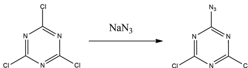
Рис. 1. Синтез 2-азида-4,6-дихлор-1,3,5-триазина
