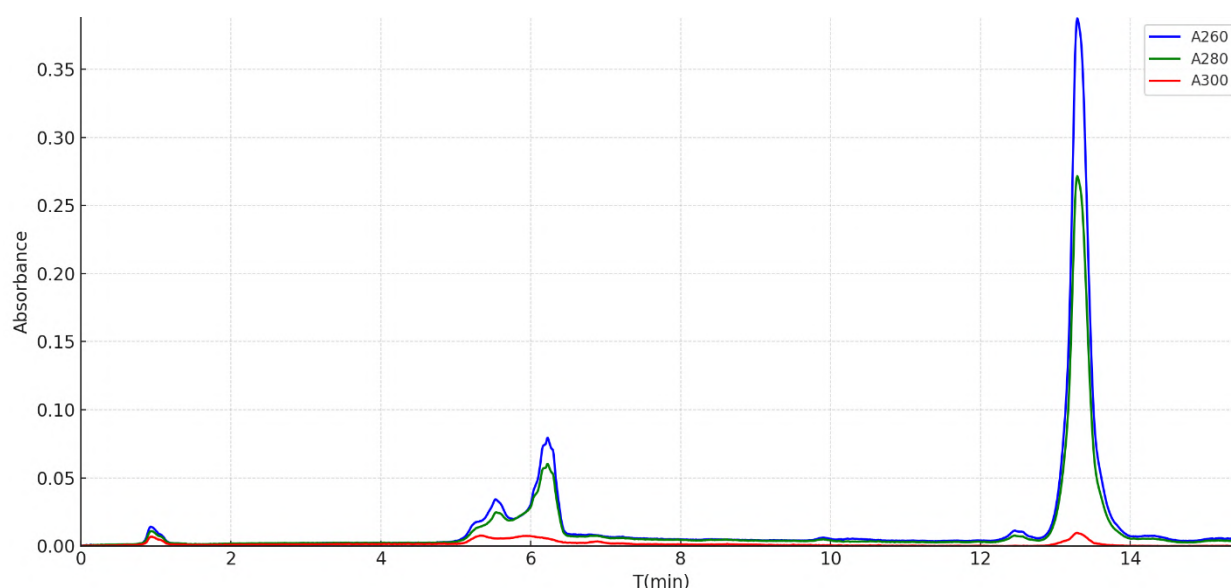
Рис. 12. Профиль ОФ ВЭЖХ реакционной смеси продуктов модификации 3-диметиламинопропиламино Т 8 -олигонуклеотида с реагентом (II) ( \lambda = 260 нм – синий, \lambda = 280 нм – зеленый, \lambda = 300 нм – красный). Градиент: 0-50% CH 3 CN (15 минут, поток 200 мкл/мин) в 0,02М водном растворе ТЕА*АсОН
