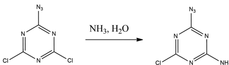
Рис. 2. Синтез 4-азида-6-хлоро-1,3,5-триазин-2-амина
