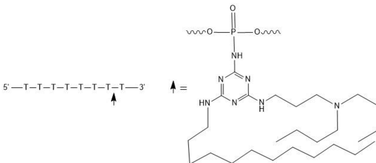
Рис. 8. N-(2-(4-додециламино-6-(3-дибутиламино)пропиламино)-1,3,5-триазин)амидофосфатная модификация
