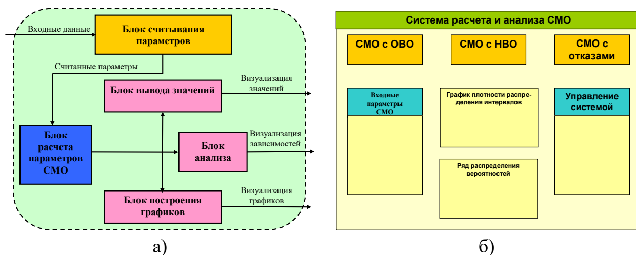
Рис. 1. Блок-схема модуля расчета параметров эффективности СМО и шаблон интерфейса
