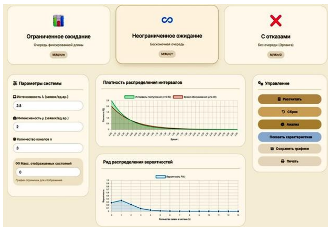
Рис. 2. Интерфейс СМО с неограниченным временем ожидания
