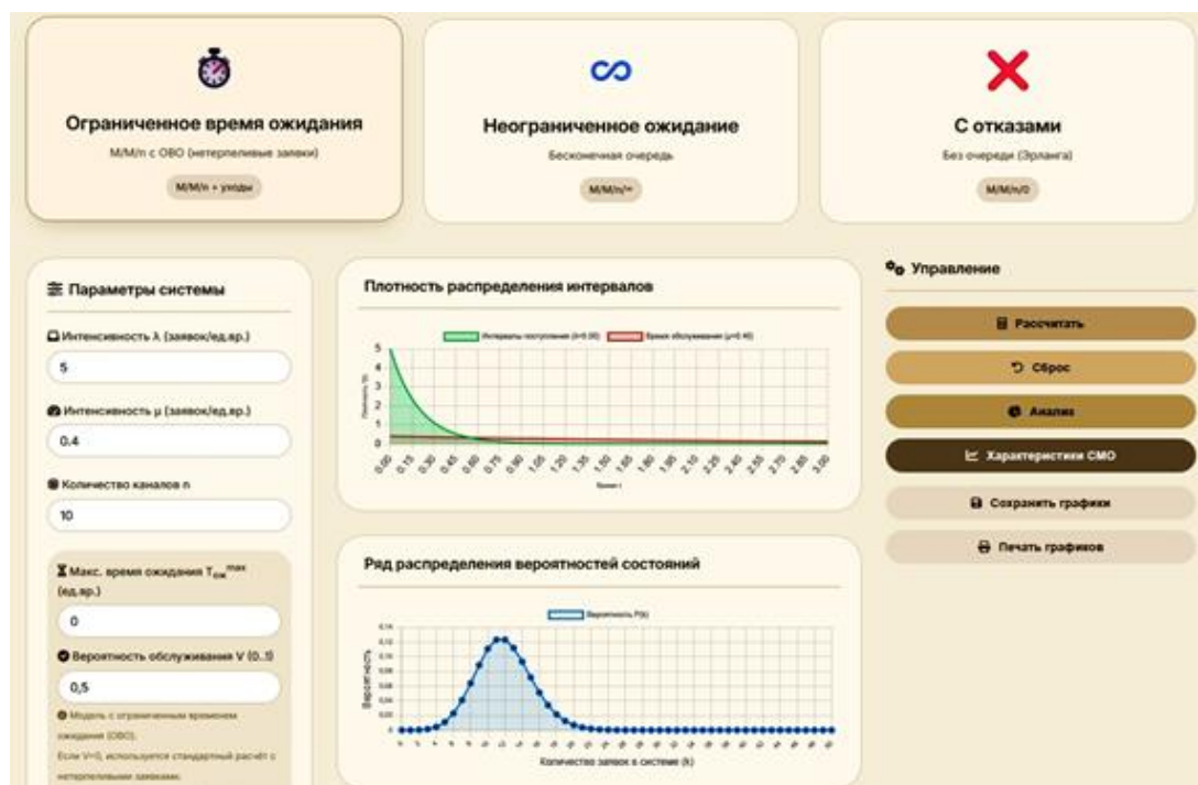
Рис. 4. Интерфейс СМО с ограниченным ожиданием
