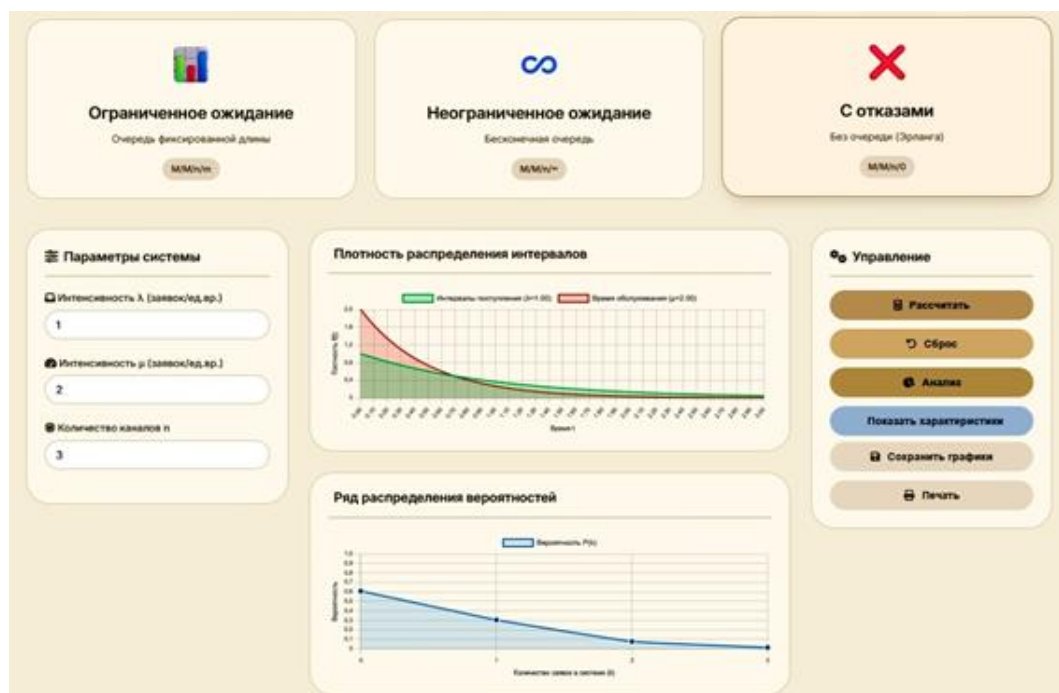
Рис. 5. Интерфейс расчета параметров СМО с отказами
