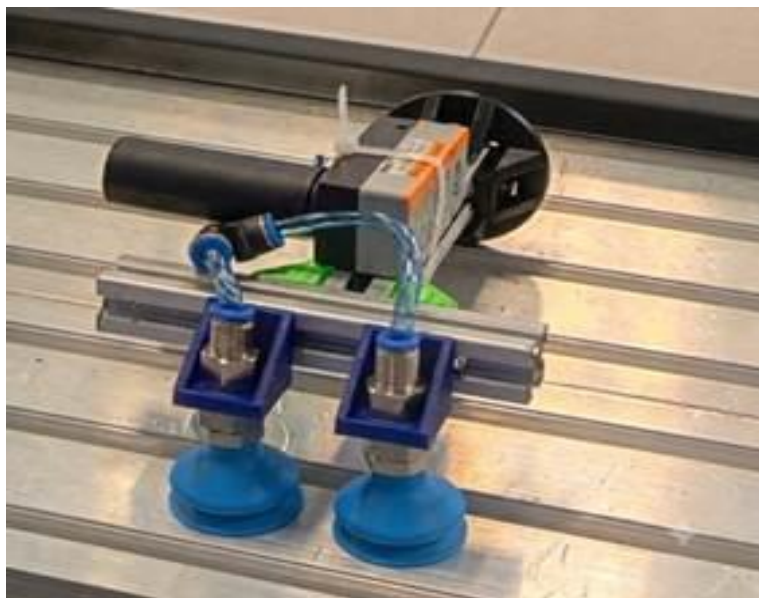
Рис. 1. Захватное устройство РТК электроэрозионной обработки
