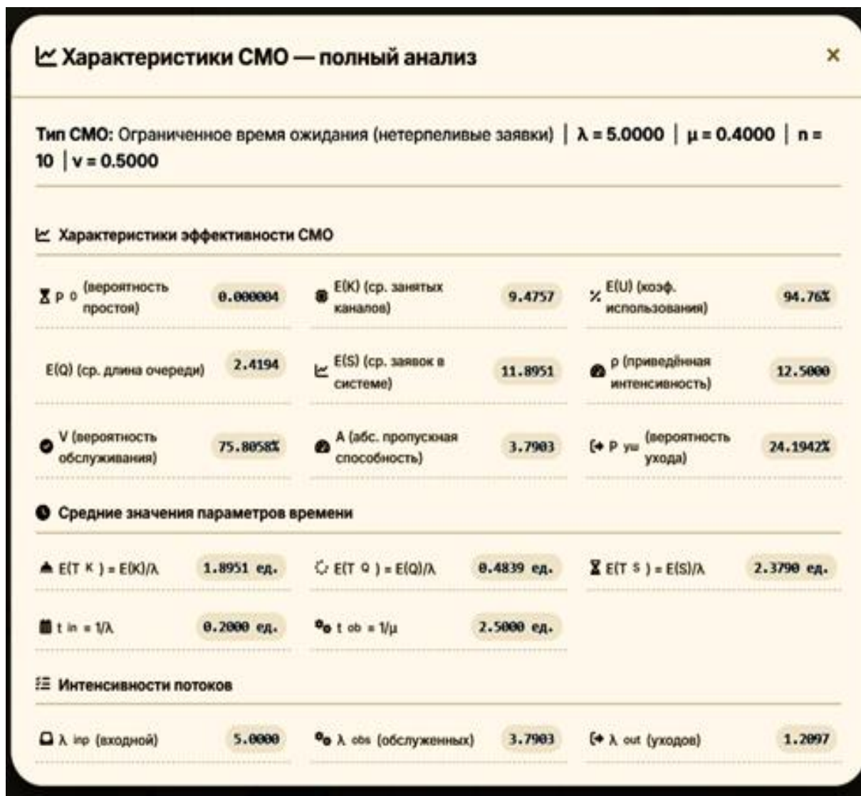
Рис. 6. Интерфейс расчета параметров СМО с отказами
