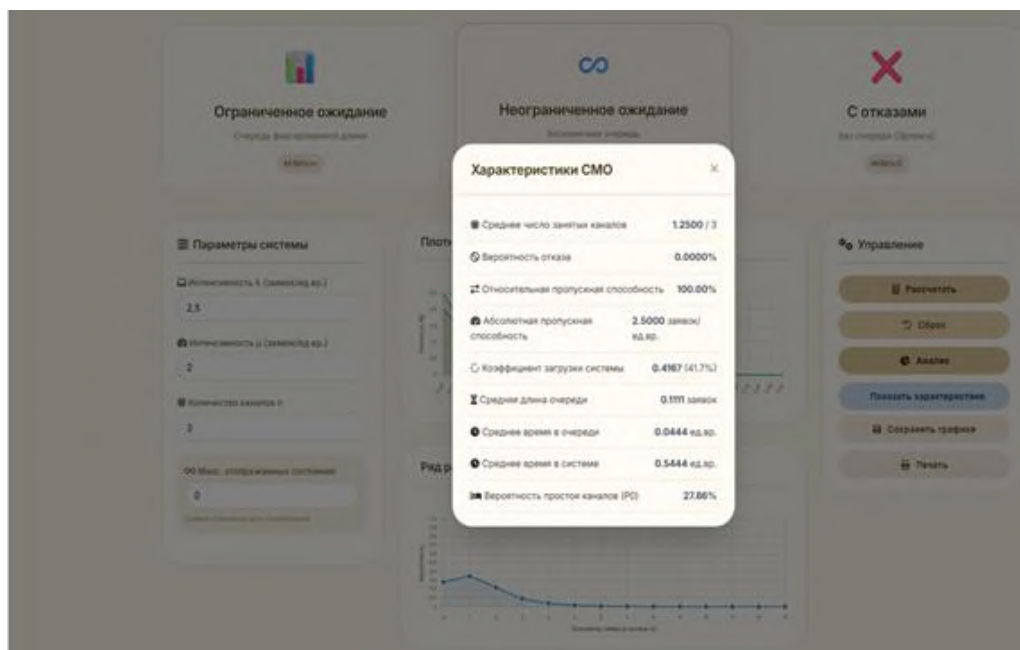
Рис. 3. Панель «Характеристики СМО»
