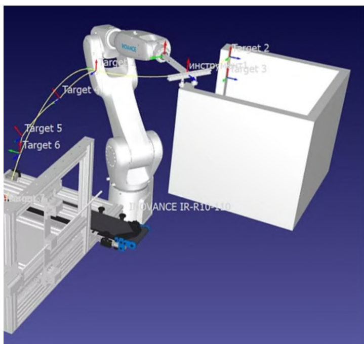
Рис. 2. Виртуальная модель РТК электроэрозионной обработки
