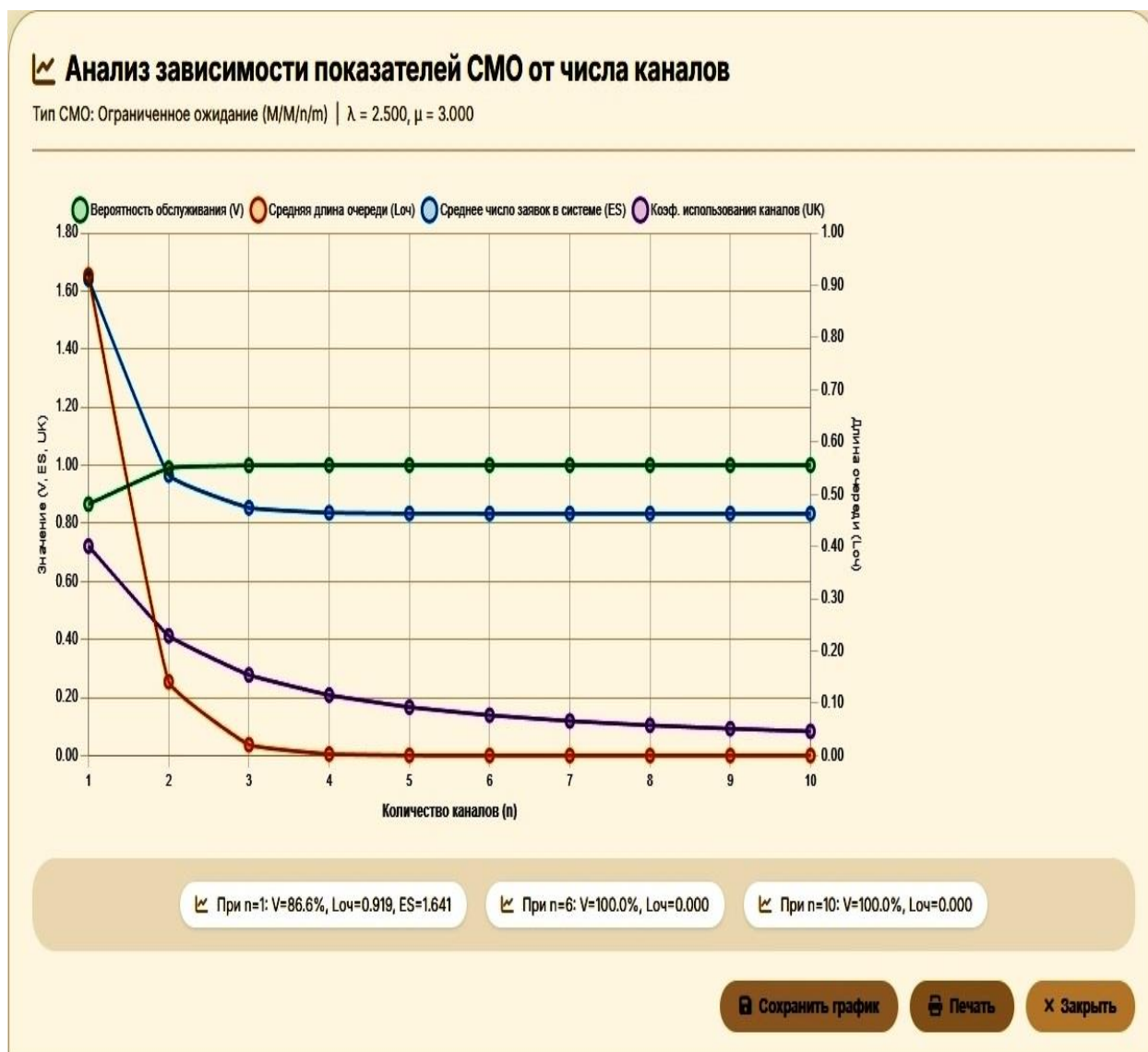
Рис. 8. Окно «Анализ» показателей эффективности от числа каналов
