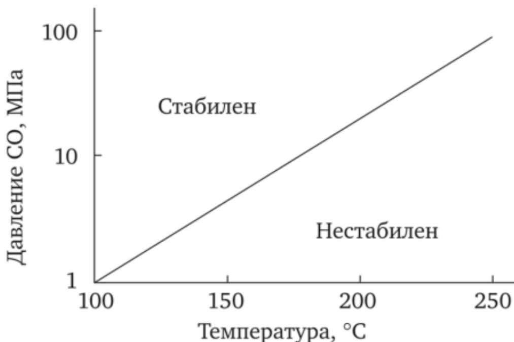
Рис. 5. Стабильность \text{NiCo(CO)}_4/\text{Co}_2(\text{CO})_8 в растворе гексана при концентрации кобальта 0,4%
