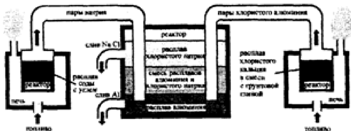
Рис. 4. Технология извлечения алюминия
