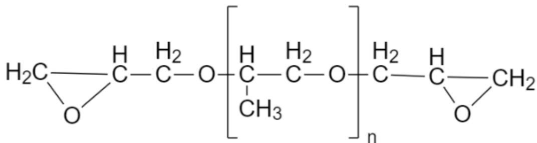
Рис. 1. Структурная формула диглицидилового эфира полиокси-пропиленгликоля
