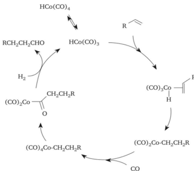
Рис. 4. Механизм гидроформилирования на кобальтовых катализаторах
