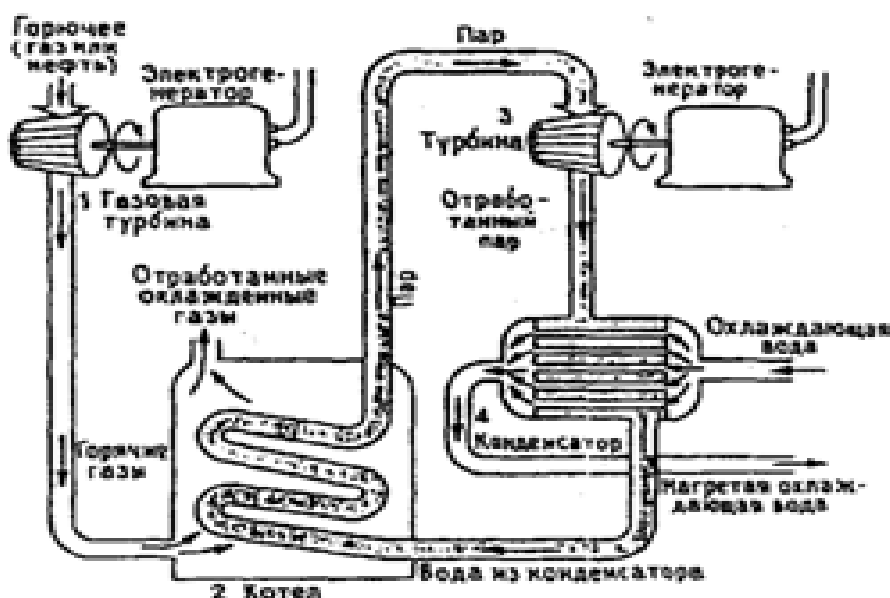
Рис. 1. Комбинированный способ получения электроэнергии
